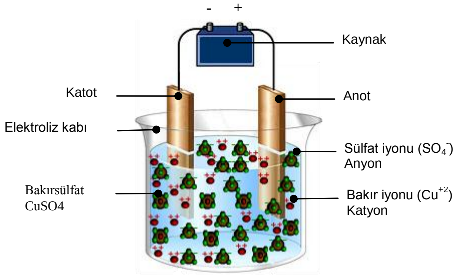
Şekil 68: Elektroliz düzeneği
