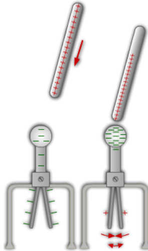
Şekil 48: Yükü elektroskop yükünden büyük olan zıt yüklü bir cismin elektroskop yapraklarına etkisi
