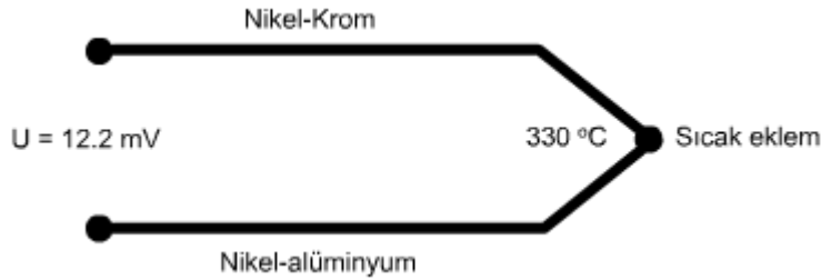
Şekil 72: Termokuplun yapısı
