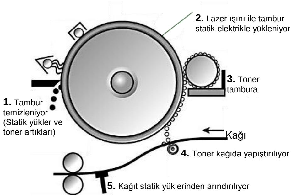
Şekil 39: Bir lazer yazıcının çalışma prensibi
