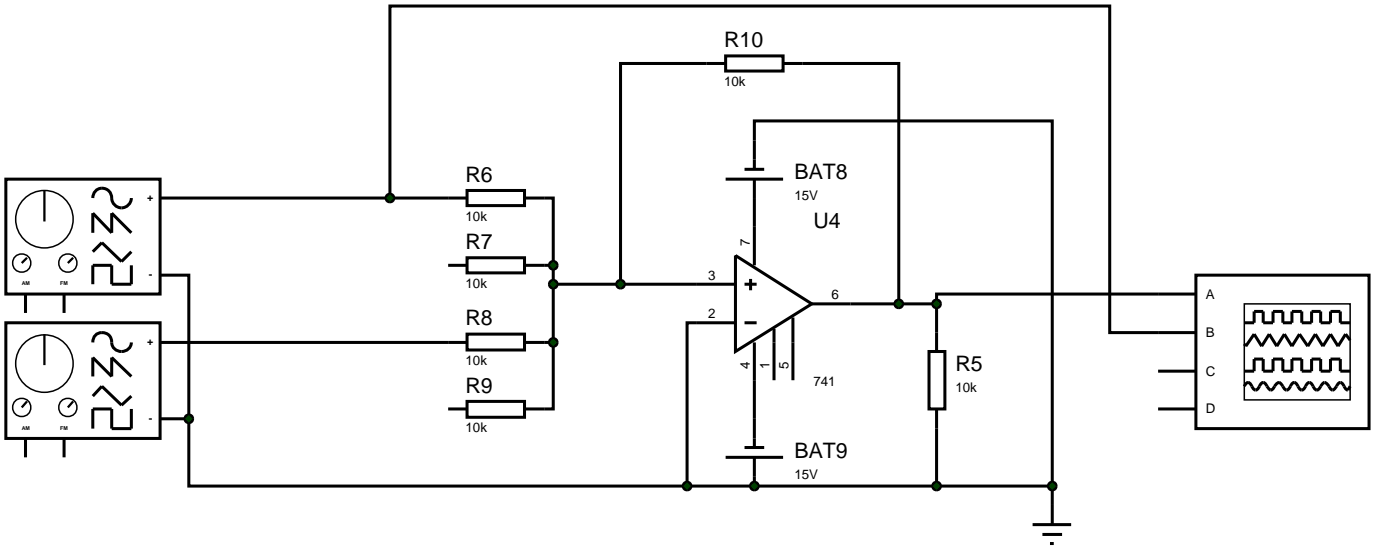
toplayici devresi
