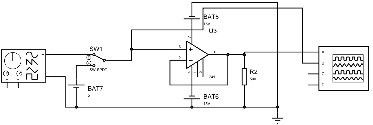
voltaj takipcisi
