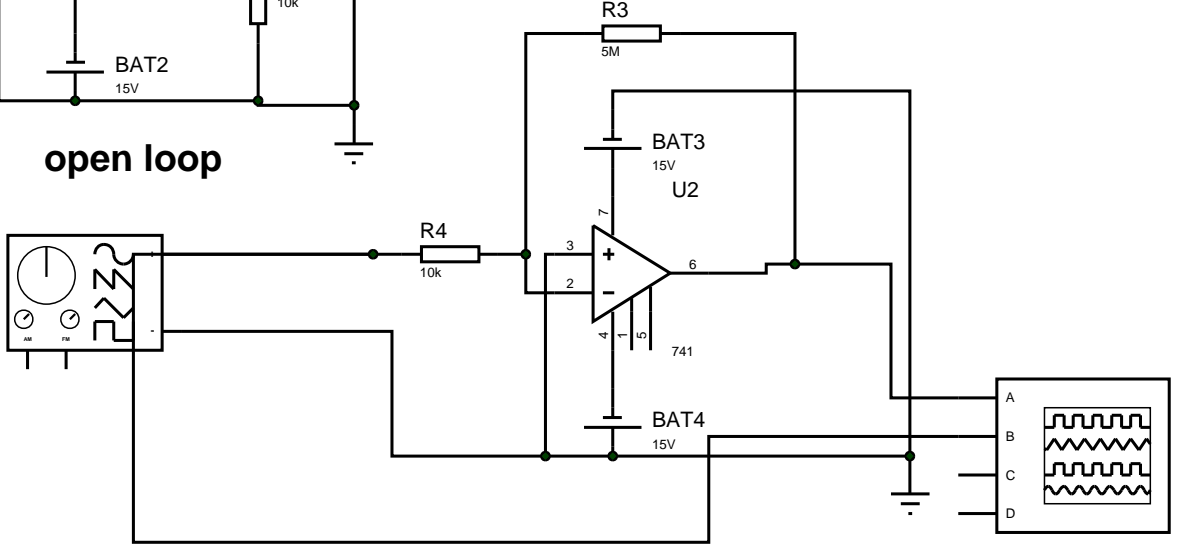
negatif geribeslemeli devre eviren yukseltec
